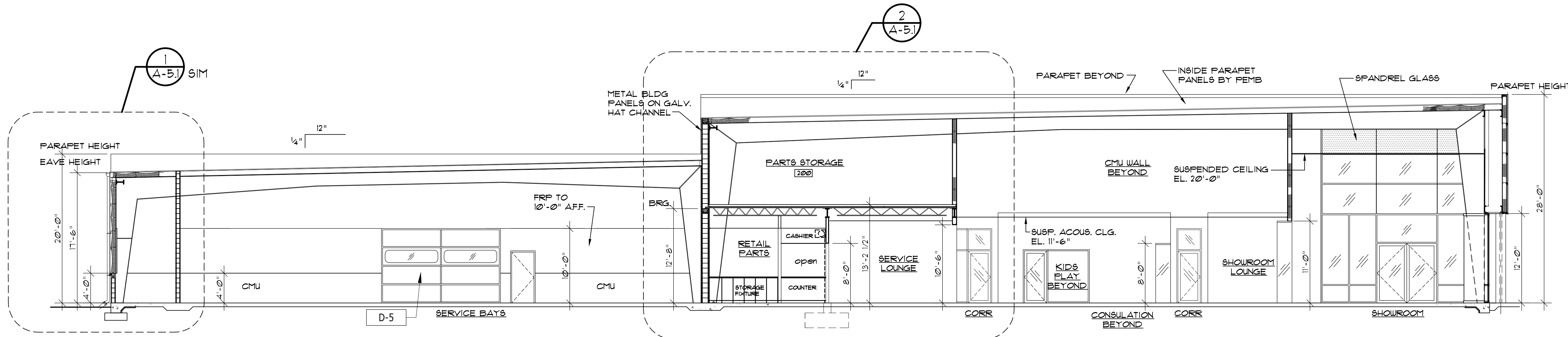
1 A-5 SCHEMATIC LONGITUDINAL BUILDING SECTION SCALE: 1/8" = 1'-0"
